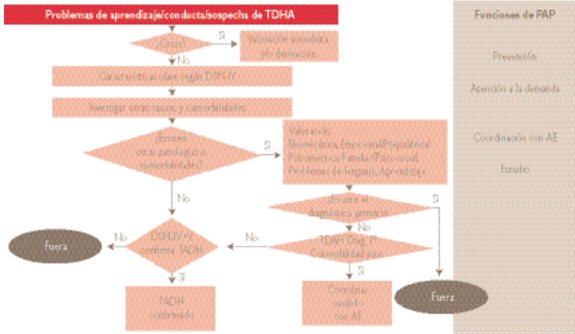
Figura I. Algoritmo 1.
