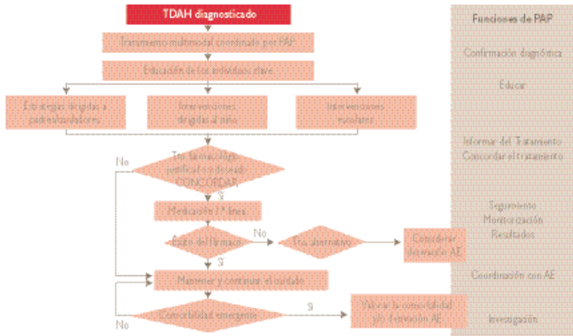
Figura II. Algoritmo 2.
